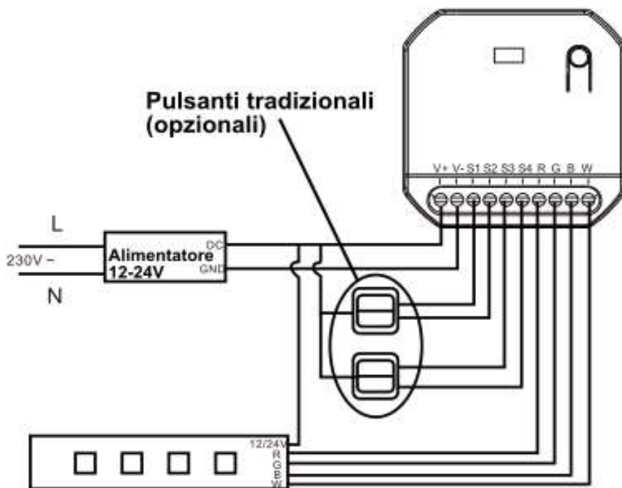
Lo schema di collegamento del 9331 – Versione precedente a Novembre 2024
