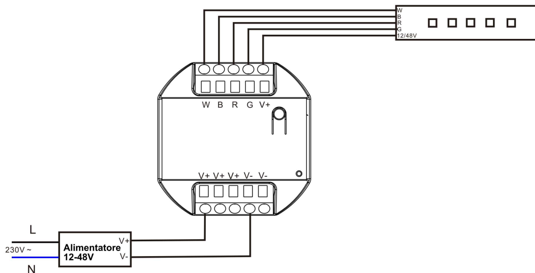
Lo schema di collegamento del 9331 – Versione da Novembre 2024
